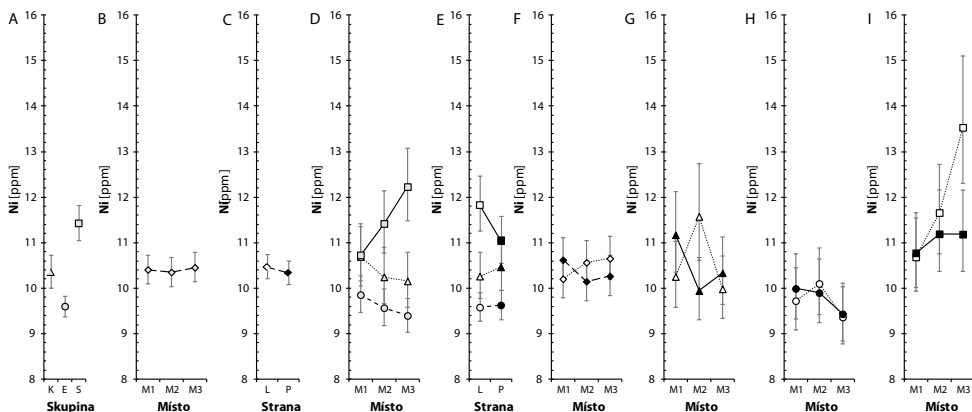
Graf 3: Vztah obsah Ni (ppm) versus skupina, místo odběru vzorků a strana odběru vzorků byl hodnocen modelem ANOVA. Symboly a označení jsou stejné jako u grafu 1.
